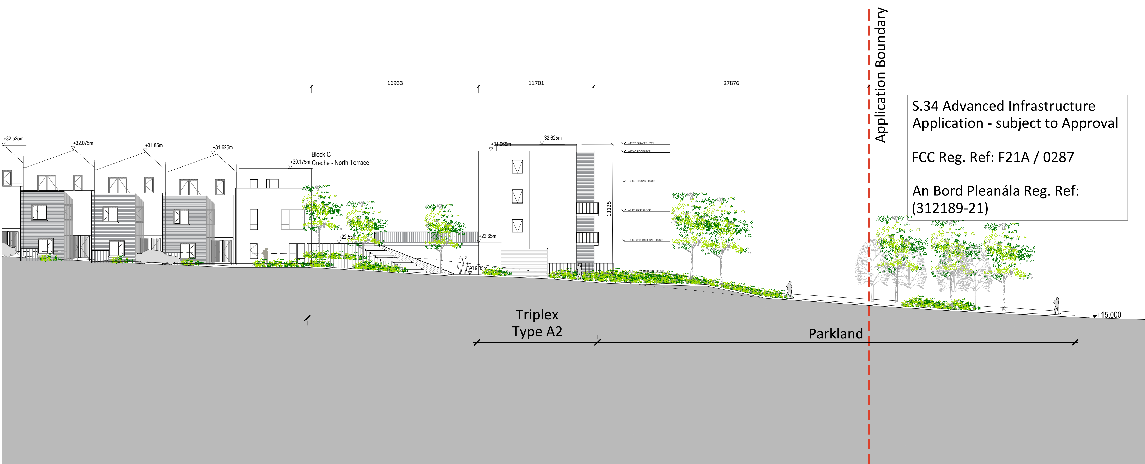
Section DD_02 Esc 1:200
